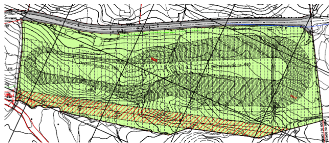
Utsnitt av reguleringsplan for riggområde og massedeponi på Støverstein
